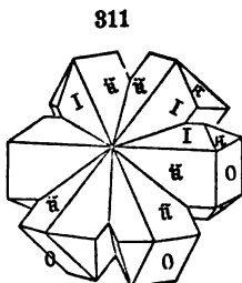
Staurolite.
